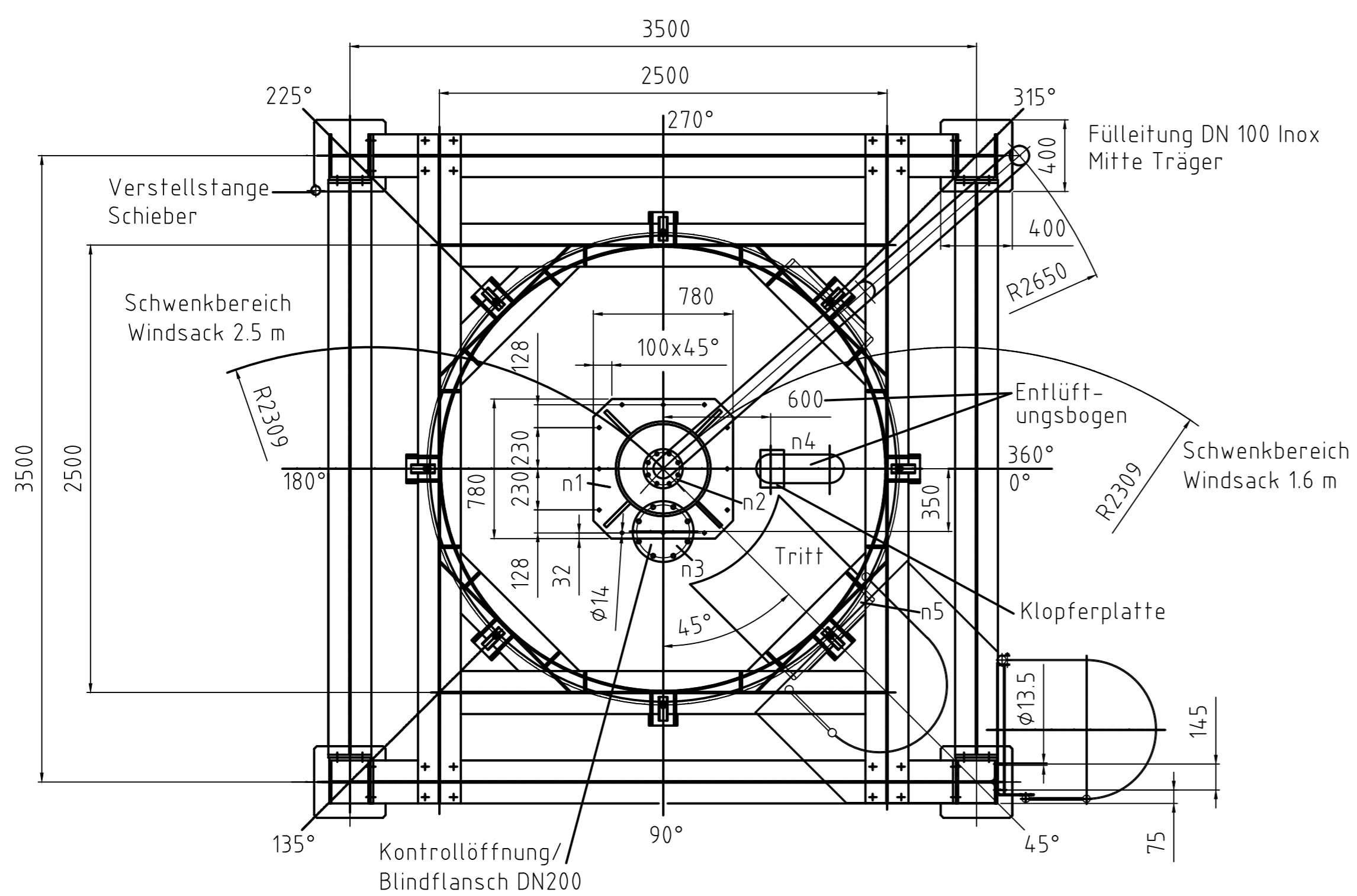
Ansicht A
