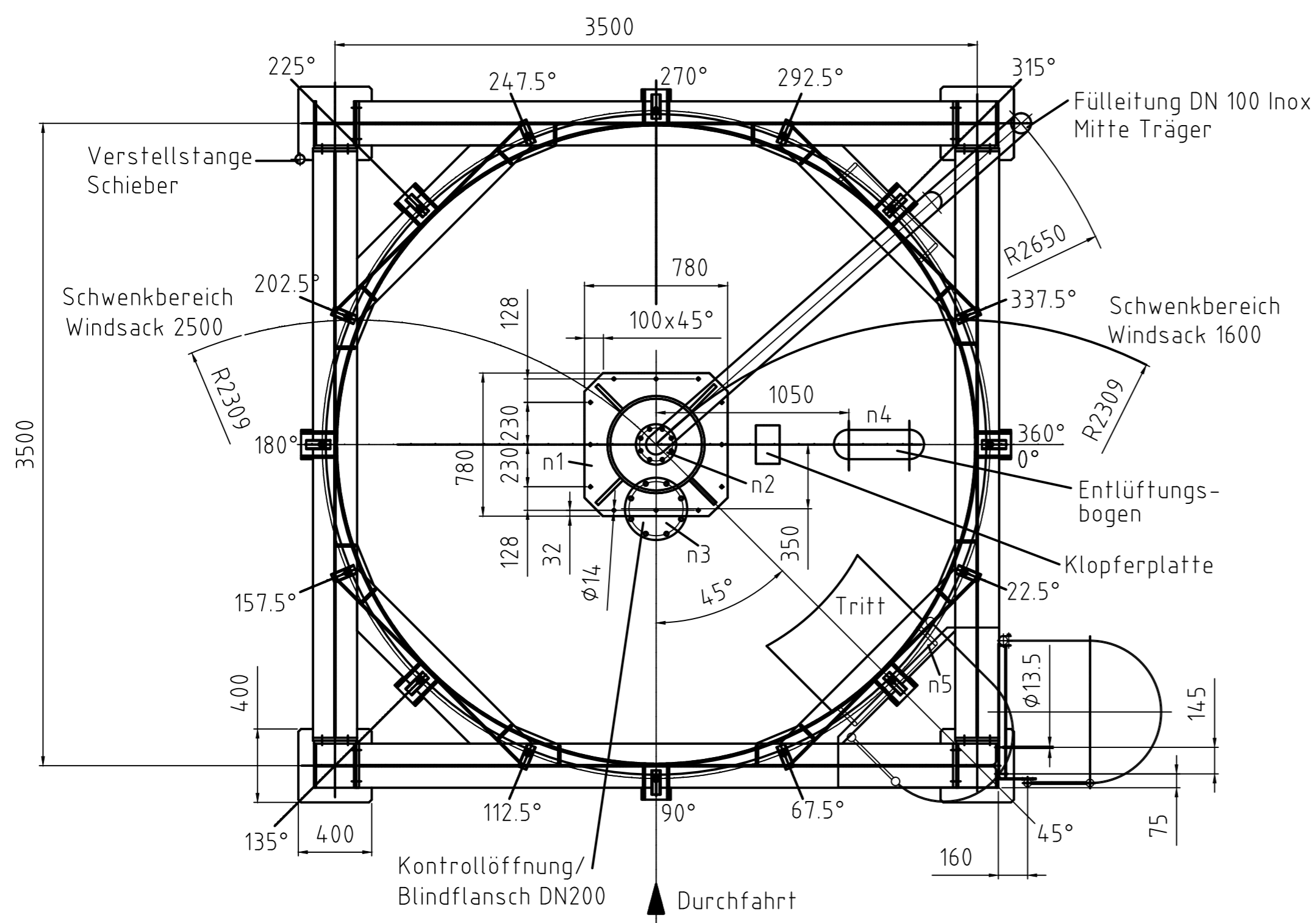
Ansicht A
