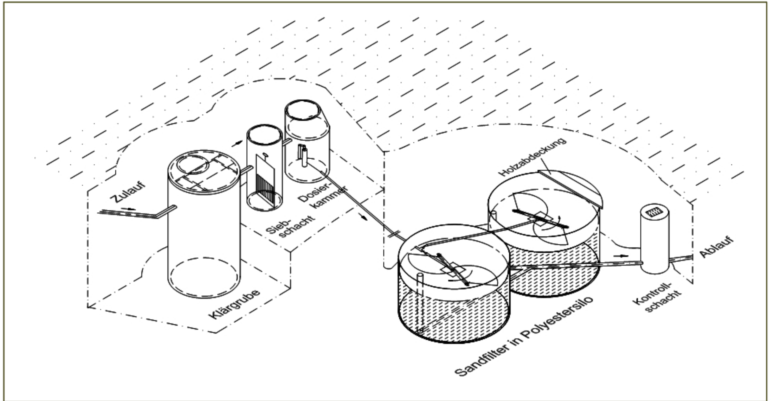
Abbildung 1: Aufbau einer Sandfilterkläranlage
